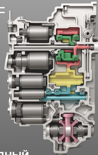
ГИБРИДНЫЙ ТРАНСМИССИОННЫЙ АГРЕГАТ
